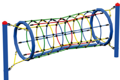
PD-4960-1 Tunelová prolézačka velikost: 3 x 0,9 m, potřebný prostor: 6,1 x 3,8 m, výška pádu: 1,3 m
