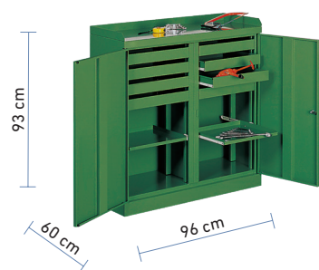
DÍLENSKÁ SKŘÍŇKA NA NÁŘADÍ, 2× DVÍŘKA, 8 VÝSUVNÝCH POLIC KÓD VÝROBKU: SZW108
