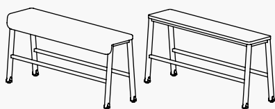
BAROVÁ LAVICE ČALOUNĚNÁ & DEKORITOVÁ (PŘEKLIŽKA) čalouněná - šířka 108 / 159 cm dekoritová - šířka: 107 / 157 cm hloubka: 45 cm výška: 77 / 76 cm
