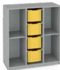
FSZ-06 korpuse z laminované dřevotřísky tl. 18 mm, plná zadní stěna, 4× zásuvka Gratnell's typu „F25“ 105x120 x4 5 cm
